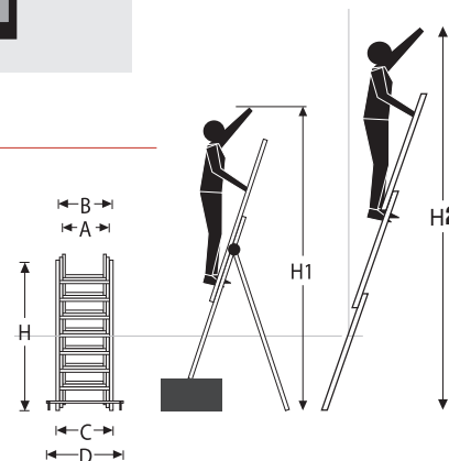
Profile o wzmacnionym przekroju 2,5 mm. Sides with 2.5 mm reinforced section.
