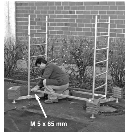
4 Podstawa rusztowania z pierwszą i drugą kondygnacją
